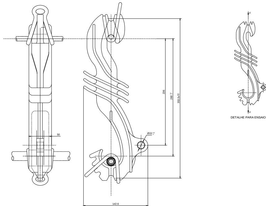
Figura 71 - Espaçador monofásico
