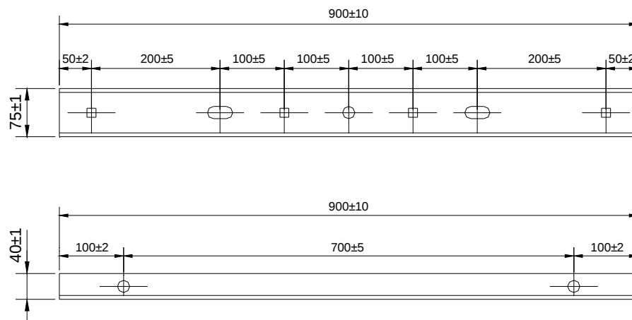
Figura 110 - Perfil U
