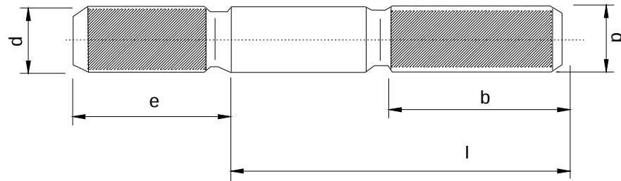
Figura 109 - Parafuso prisioneiro
