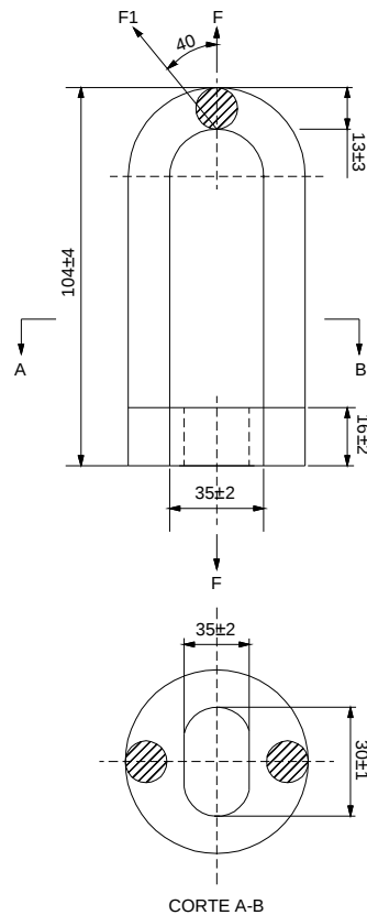
Figura 104 - Olhal para parafuso
