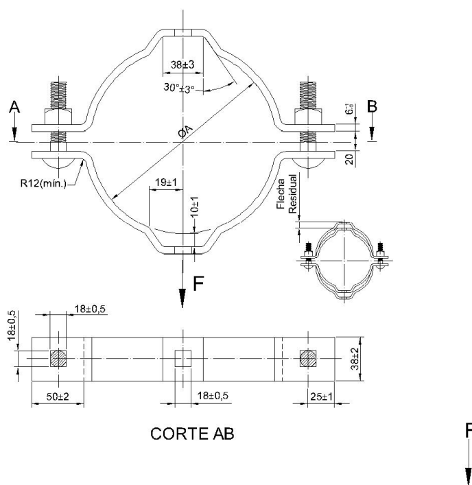
Figura 35 - Cinta para poste circular
