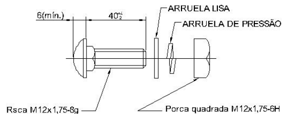
Figura 134 - Suporte T
