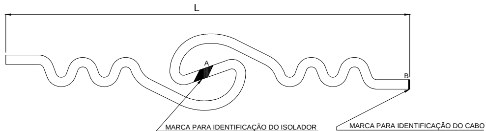
Figura 92 - Laço pré-formado de topo
