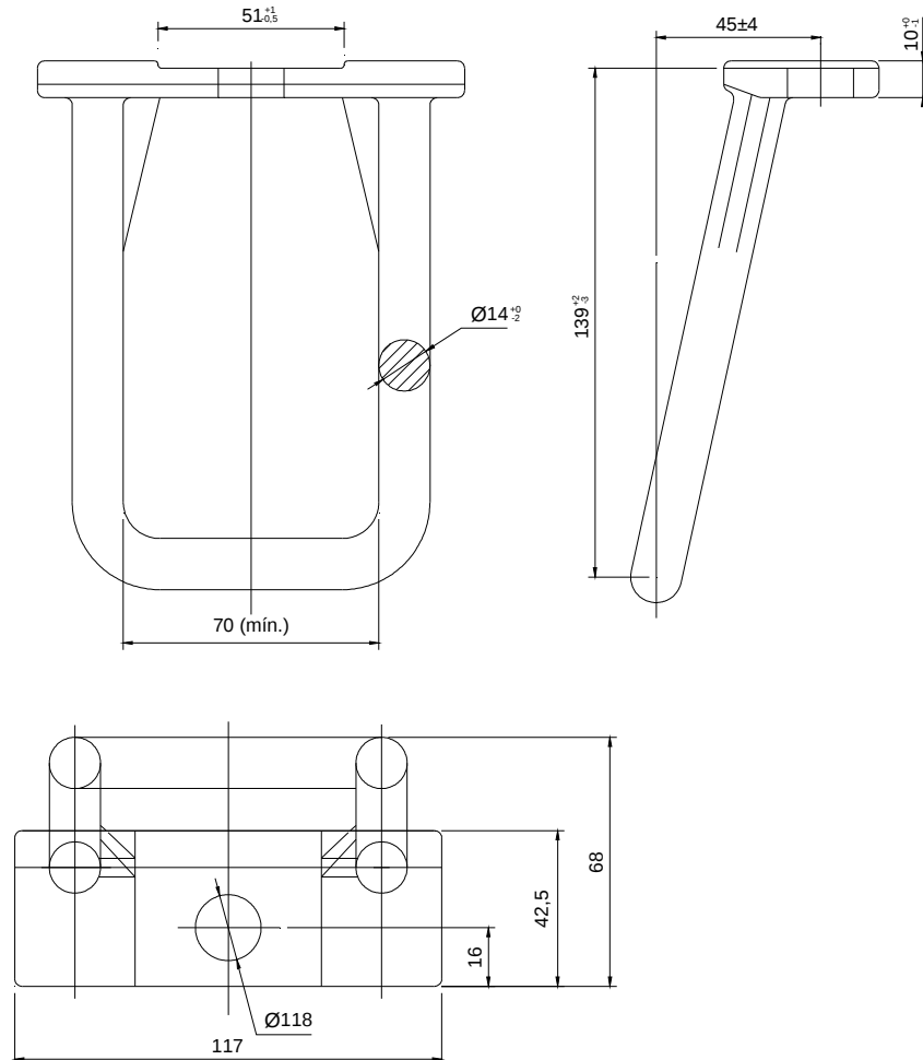
Figura 73 - Estribo para braço tipo L
