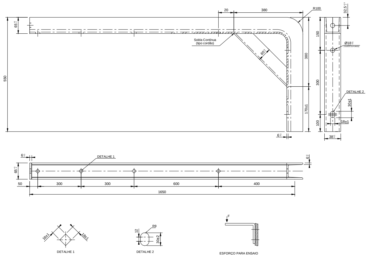
Figura 123 - Suporte afastador
