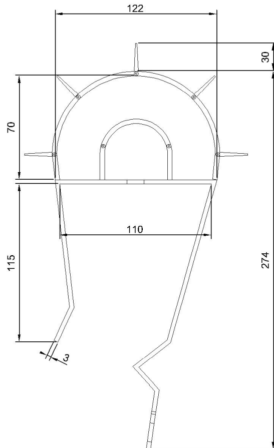
Figura 85 - Inibidor de ninho de pássaros
