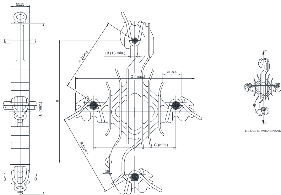
Figura 70 - Espaçador losangular
