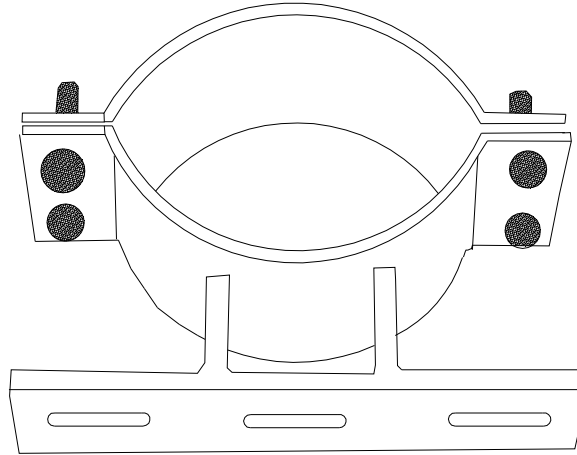
Figura 128 Suporte para equipamento tipo III
