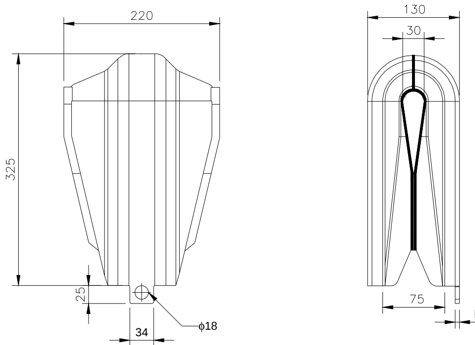
Figura 26 - Capa protetora polimérica para grampo de linha viva
