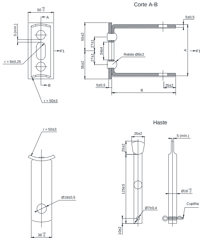
Figura 11 - Armação secundária tipo pesada de um estribo
