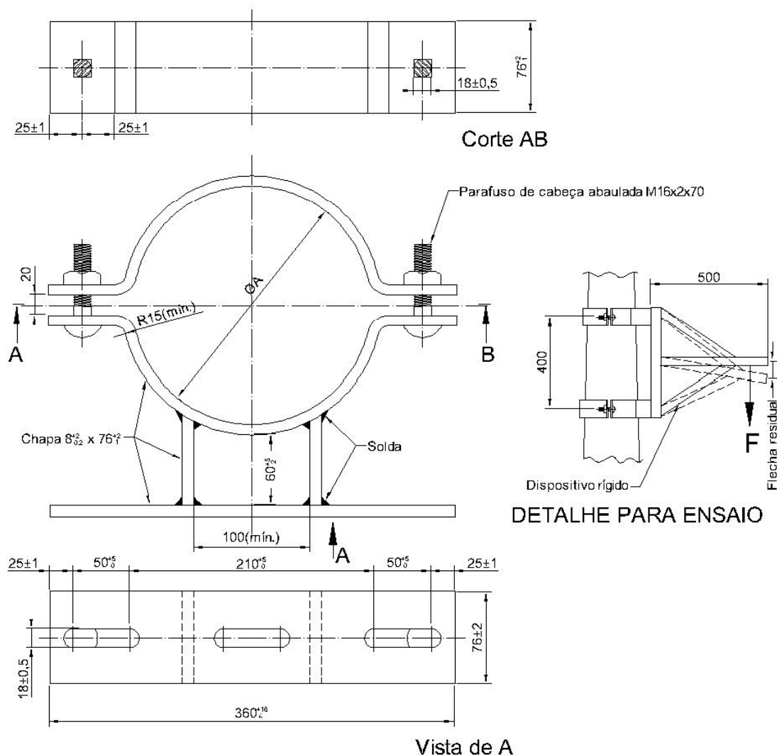
Figura 132 - Suporte para transformador - Poste circular de concreto
