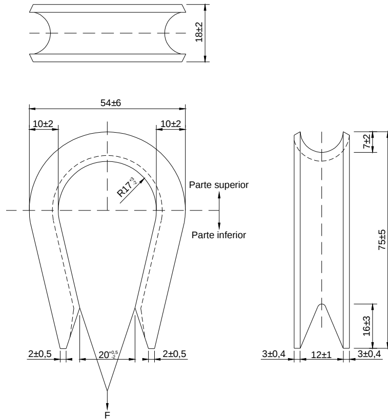
Figura 121 - Sapatilha
