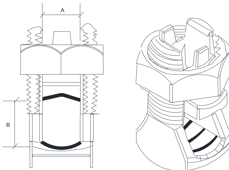
Figura 43 - Conector de parafuso fendido
