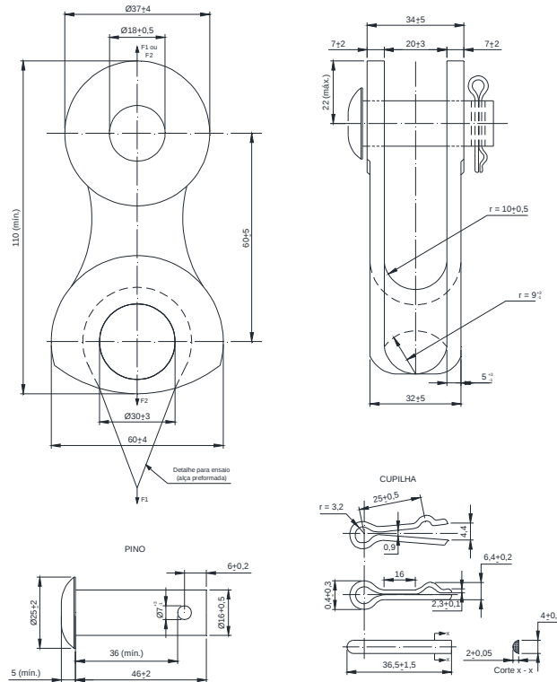
Figura 98 - Manilha sapatilha
