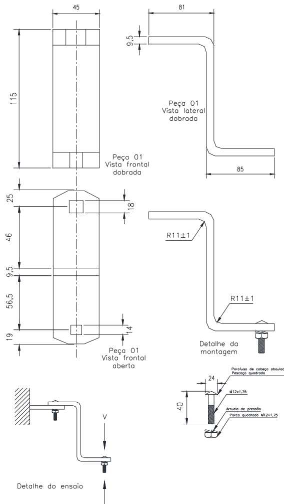
Figura 136 - Suporte Z
