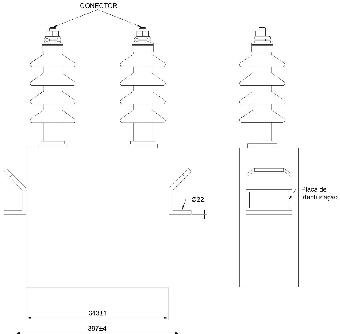
Figura 29 - Célula capacitiva
