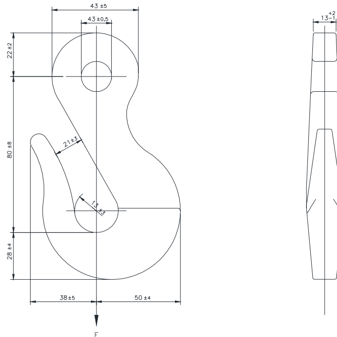
Figura 78 - Gancho olhal
