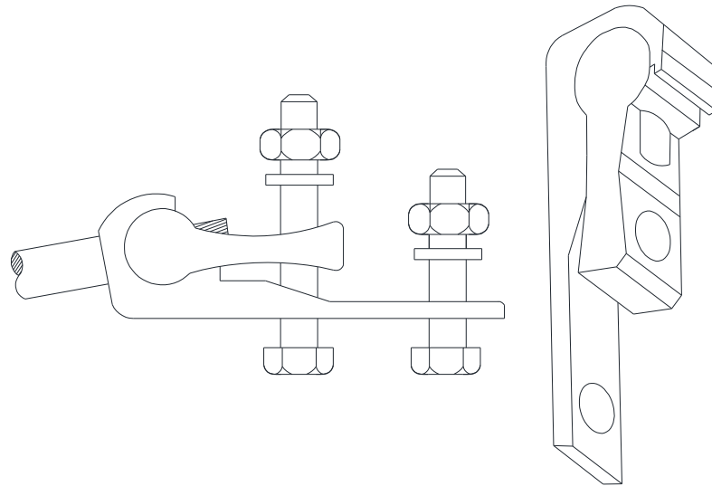
Figura 51 - Conector terminal de estrangulamento
