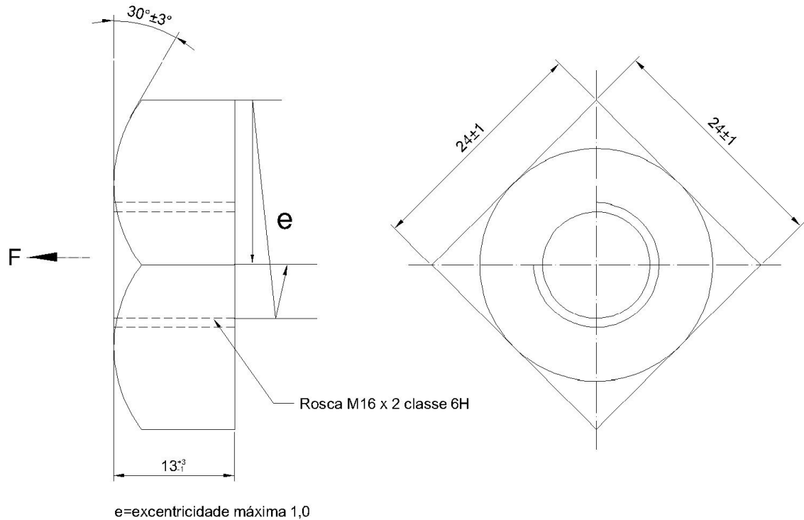
Figura 115 - Porca quadrada
