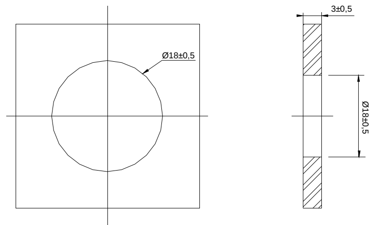
Figura 14 - Arruela quadrada
