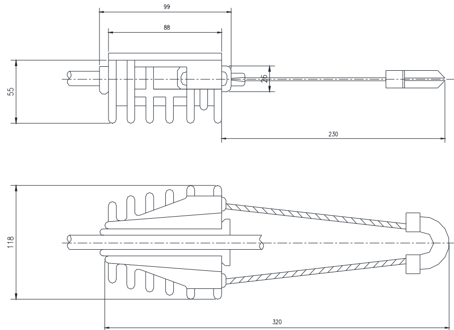
Figura 79 - Grampo de ancoragem
