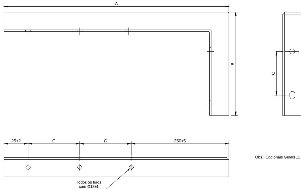
Figura 127 - Suporte horizontal
