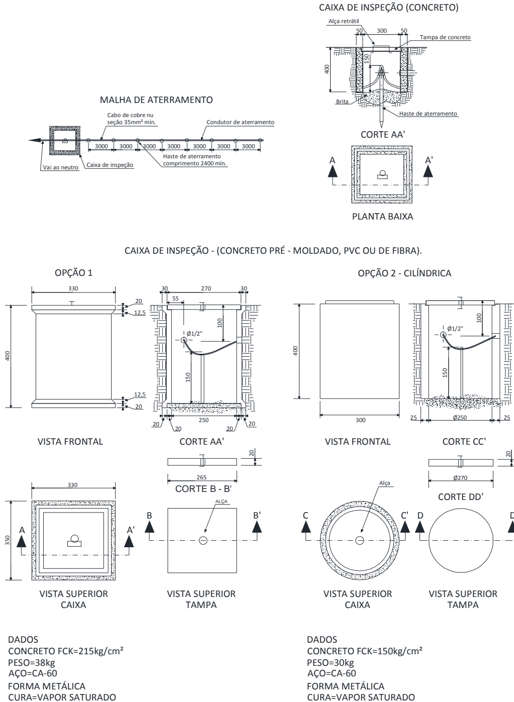
Figura 40 - Aterramento
